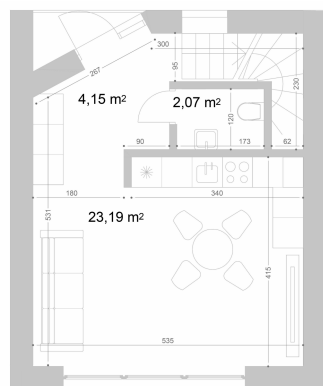
2 AUKŠTAS
